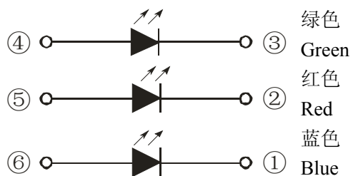
极性 Polarity
