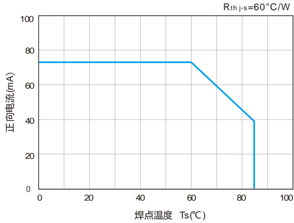
正向电流降额曲线
