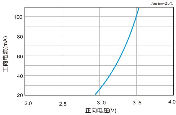
伏安特性
