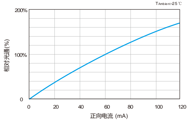
相对光通与正向电流特性
