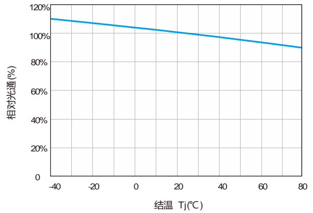
光通随结温变化曲线
