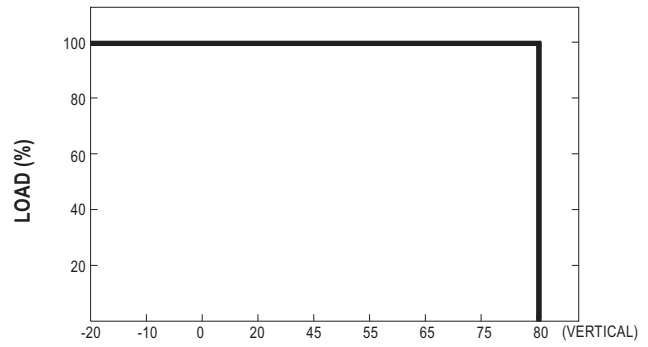
Tcase (°C)
