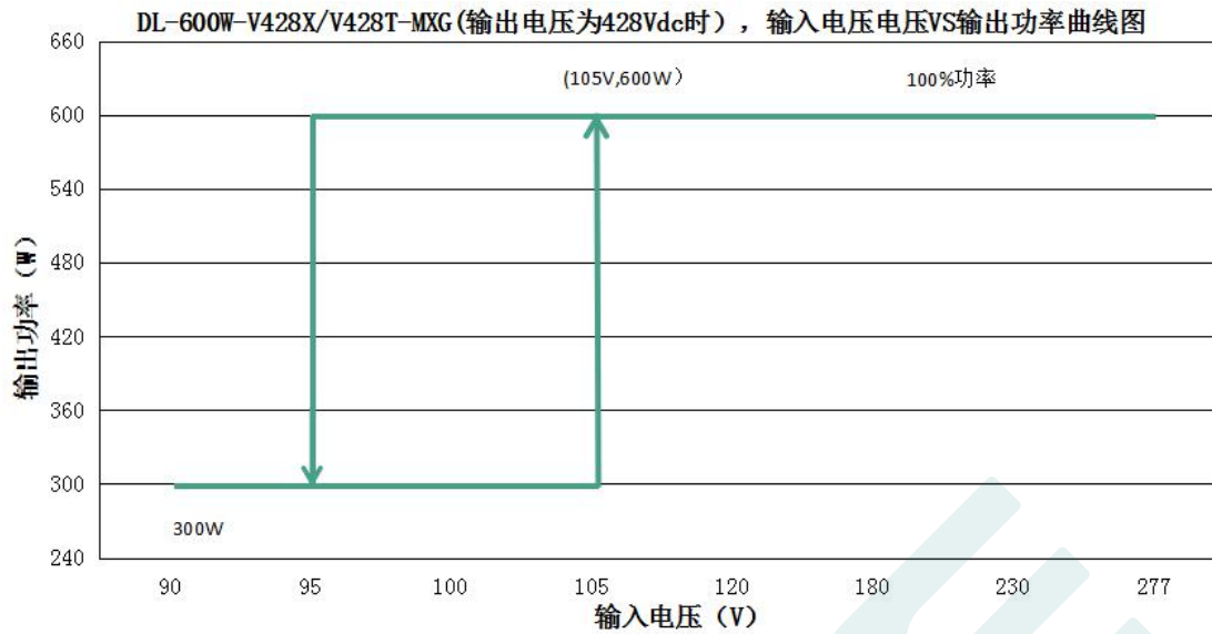
DL-600W-V428X/V428T-MXG(输出电压为 428Vdc 时, 不同输入电压对应的额定输出电流值和输出功率)
