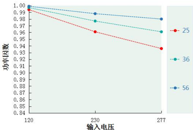
功率因素 VS 输入电压 DL-600W-V56X/T-MXG
