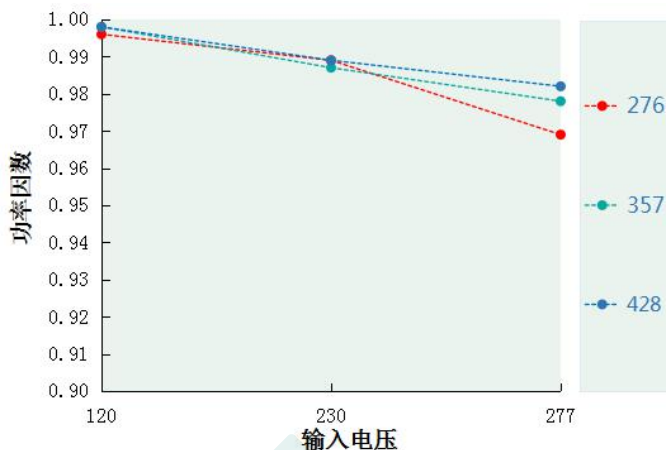
功率因素 VS 输入电压 DL-600W-V428X/T-MXG
