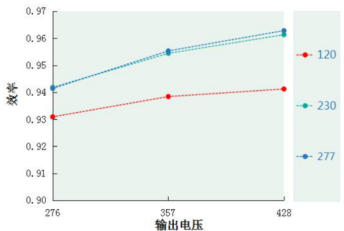
效率 VS 输出电压 DL-600W-V428X/T-MXG
