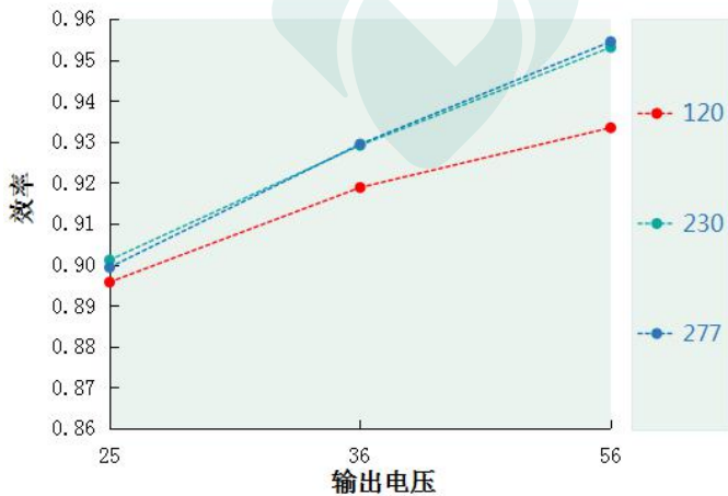
效率 VS 输出电压 DL-600W-V56X/T-MXG
