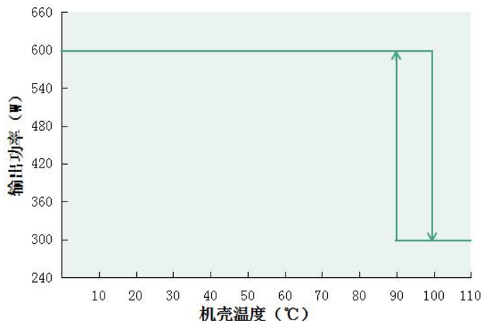
输出功率 VS 机壳温度 (DL-600W-MXG)
