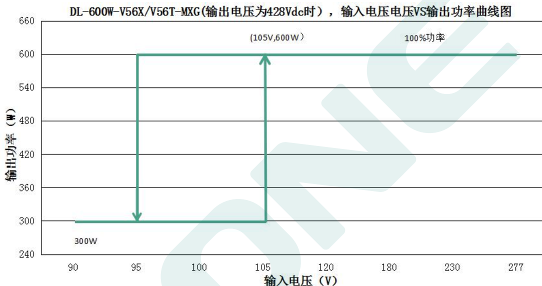
DL-600W-V56X/V56T-MXG(输出电压为 56Vdc 时, 不同输入电压对应的额定输出电流值和输出功率)
