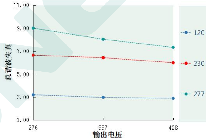
总谐波失真 VS 输出电压 DL-600W-V428X/T-MXG
