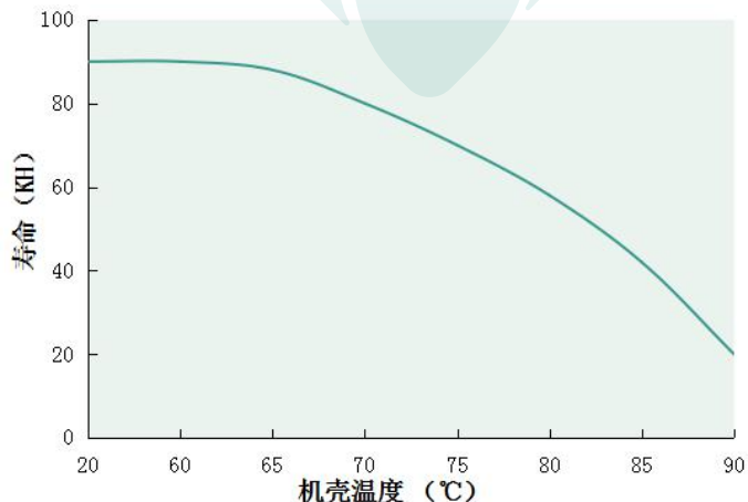
Tc VS 寿命 (DL-600W-MXG)
