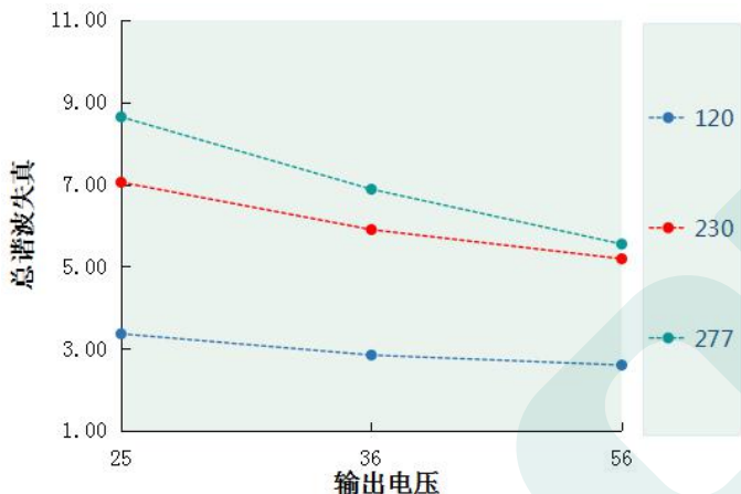
总谐波失真 VS 输出电压 DL-600W-V56X/T-MXG
