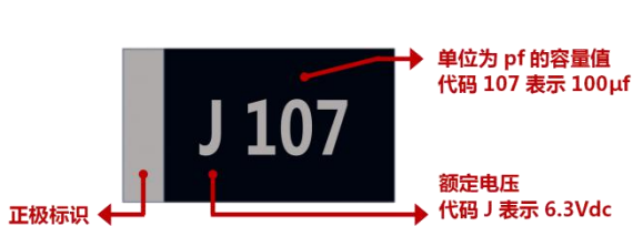
图 1 规格为 6.3V100B 的产品打印标识图示
