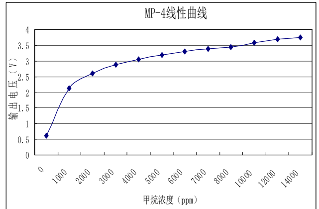
Fig6. Linear curve
