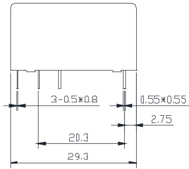
安装图
